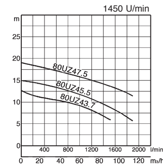
Kanalarbeiten: UZ-Serie Seite 9 Freistromlaufwerk mit großem Durchgang
